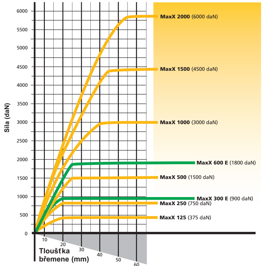
Křivka: síla/tloušťka
